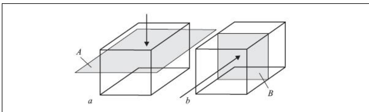
Figura 2 – Direção da circulação do gás de resfriamento: a) forno com câmara de seção retangular; b) forno com seção cilíndrica.
