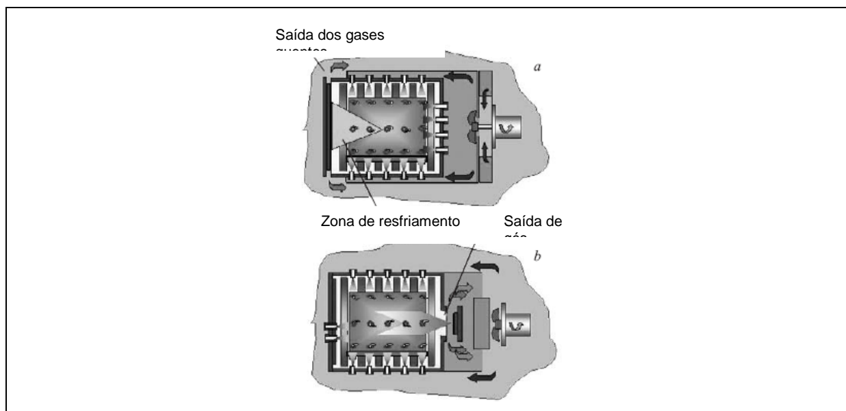
Figura 4 – Diagrama do fluxo de gás na câmara a) convencional; e b) câmara de projeto SW
